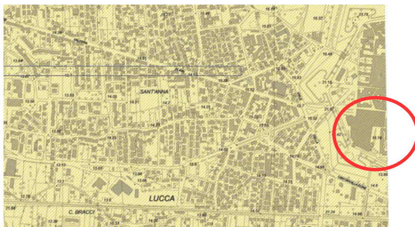
Figura 22 - Estratto dell'Elaborato PS.9 "Carta della pericolosità sismica"- Variante al RU per adeguamento alla normativa sismica - 15.05.2007
