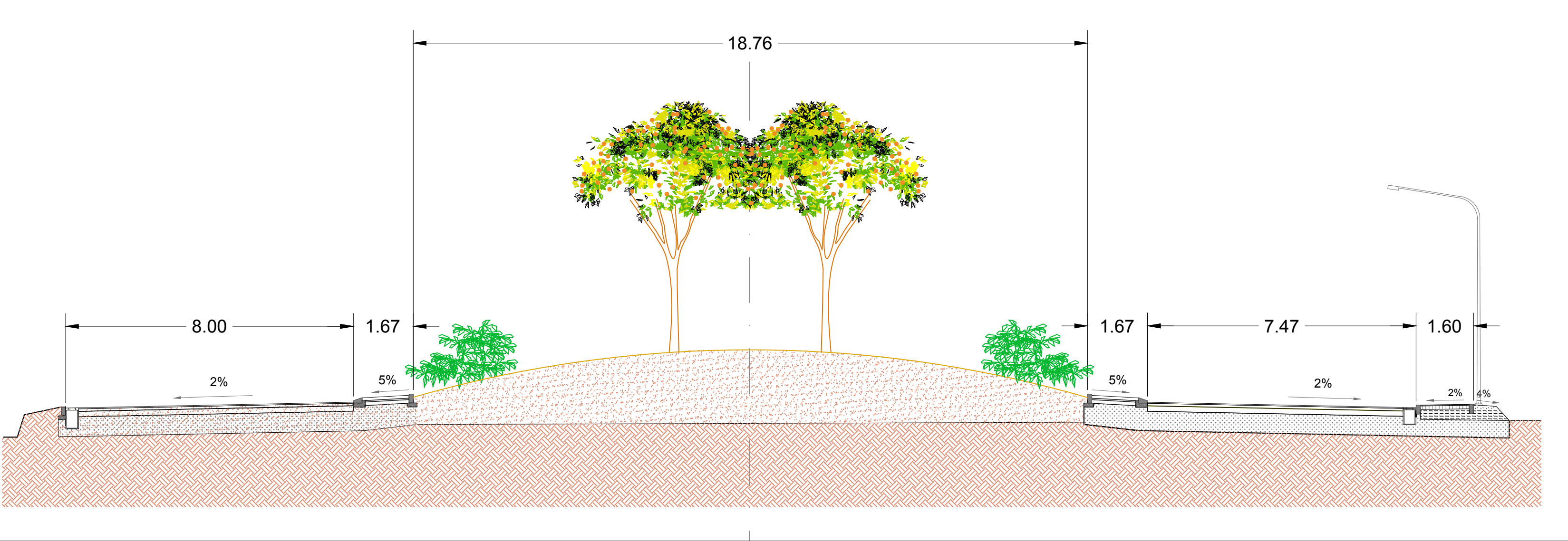
SEZIONE 1 - ROTATORIA VIA DELL'ACQUACALDA
