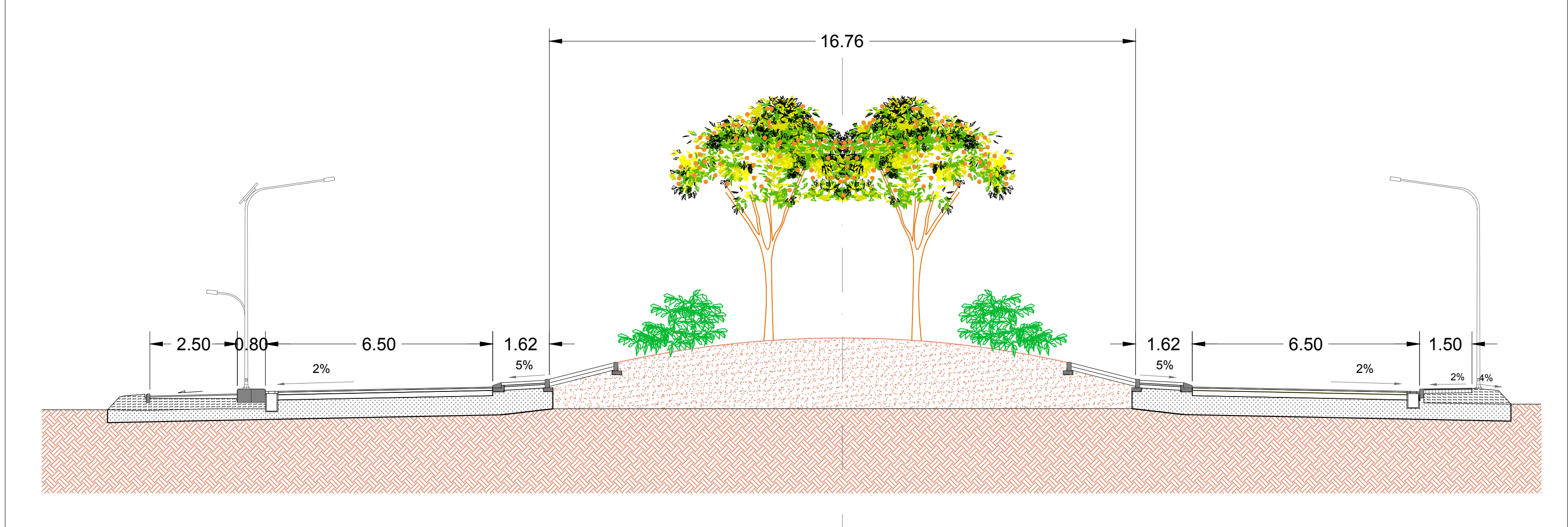
SEZIONE 39 - ROTATORIA VIA SS. ANNUNZIATA
