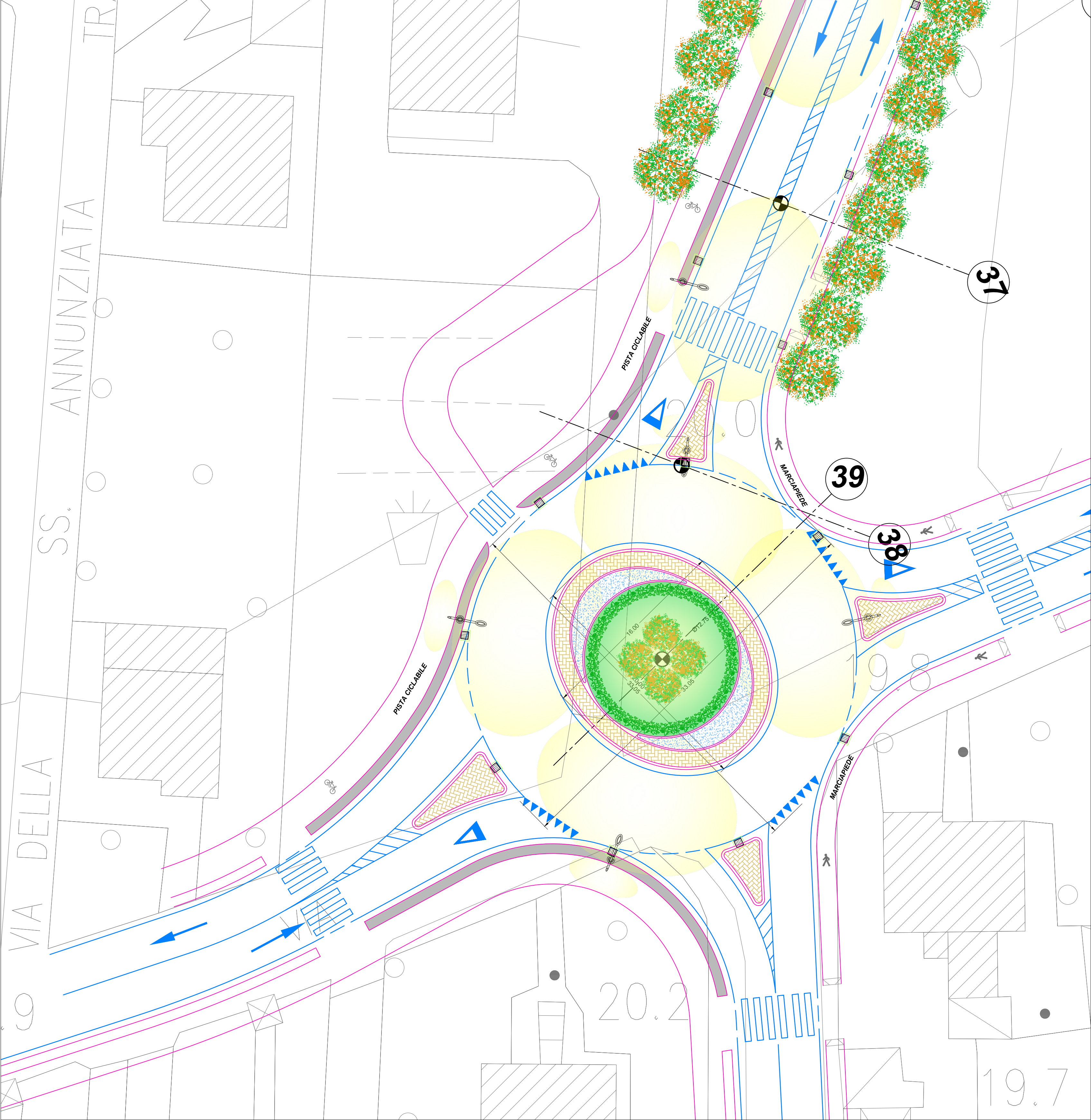
ROTATORIA VIA SS. ANNUNZIATA
