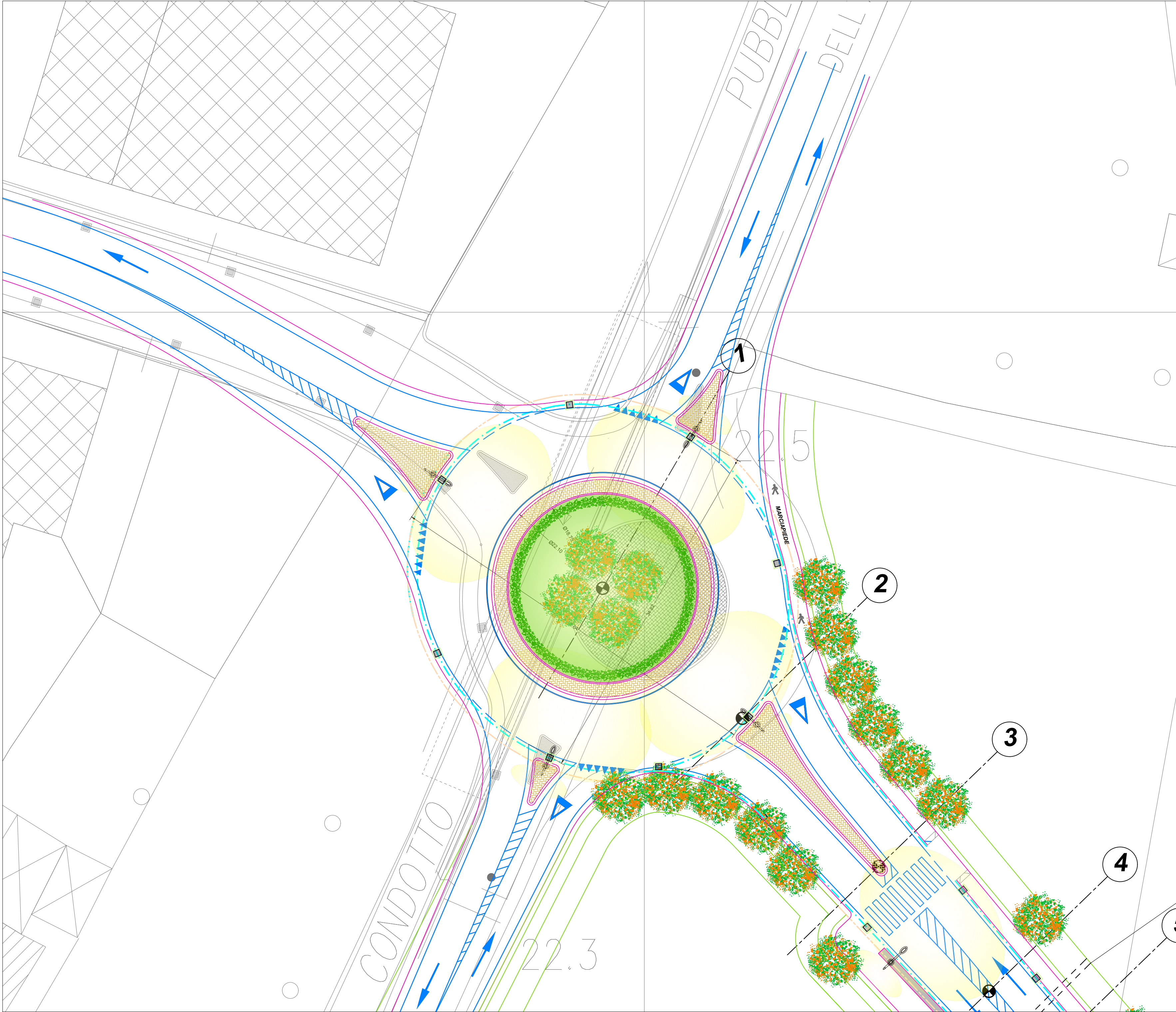
ROTATORIA VIA DELL'ACQUACALDA
